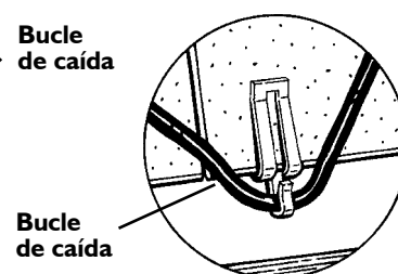
Figura 14. Sujete las pinzas a las tejas del techo sin los canalones
