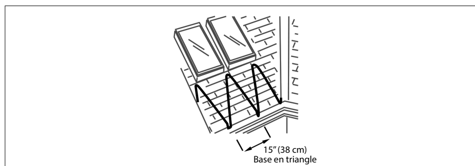
Figure 3. Configuration de la ligne d'horizon
